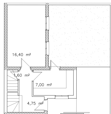
PLANTA BAJA
