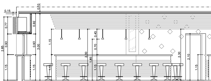
SECCION LONGITUDINAL A BARRA
