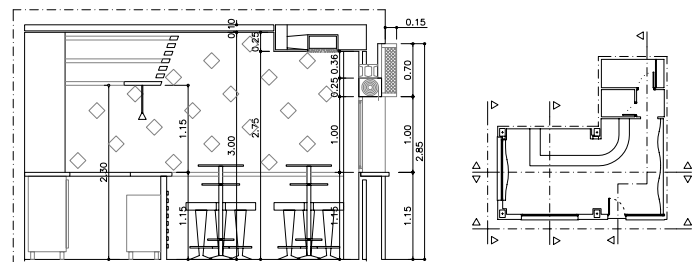
SECCION TRANSVERSAL A MEDIANERA
