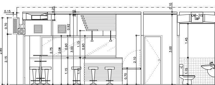
SECCION TRANSVERSAL A FACHADA
