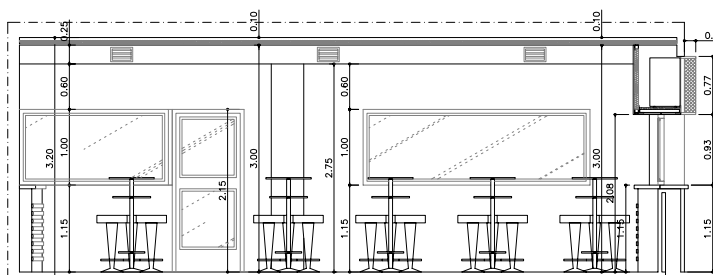
SECCION LONGITUDINAL A FACHADA
