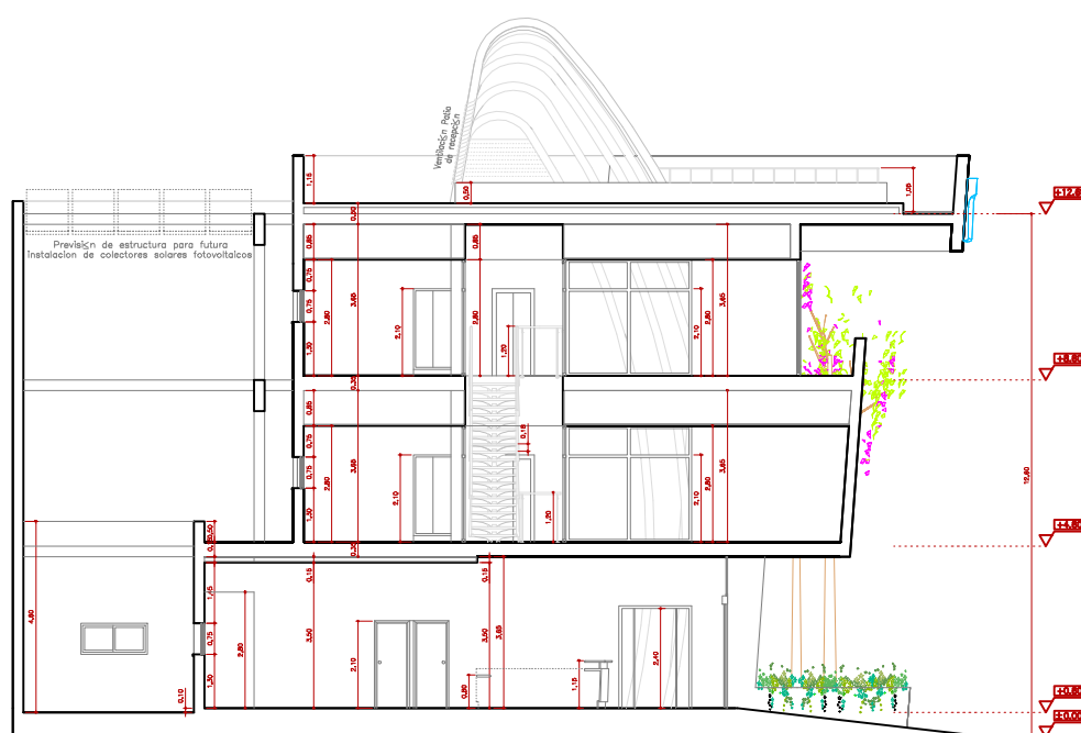
SECCION LONGITUDINAL 3
